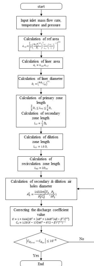
شکل (۱): نمودار گردش طراحی محفظه [۸]
