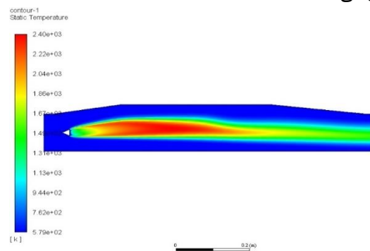
شکل (۸): نمودار دمای محفظه احتراق بدون ورود هوای ثانویه
