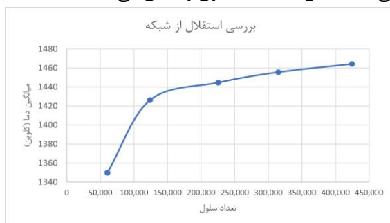
شکل (۴): میانگین دمای محفظه در شبکه‌بندی‌های
