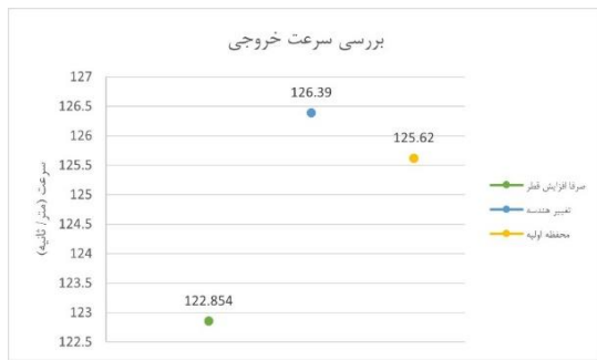
شکل (۱۳): مقایسه سرعت خروجی در محفظه‌های با ابعاد
