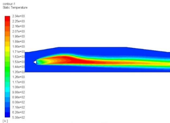
شکل (۳): کران نمای دمای محفظه
