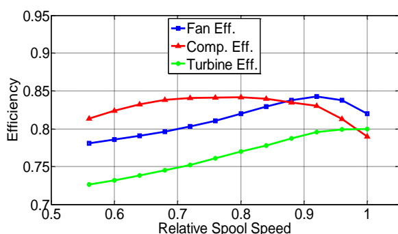
شکل (۱۴): تغییر بازده اجزای موتور در دورهای مختلف
