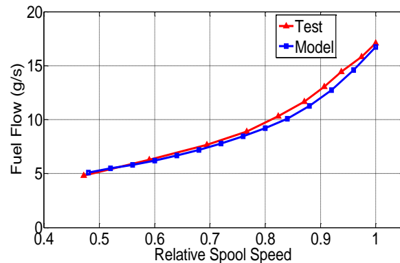
شکل (۳): سوخت موتور پایه برحسب دور نسبی شفت
