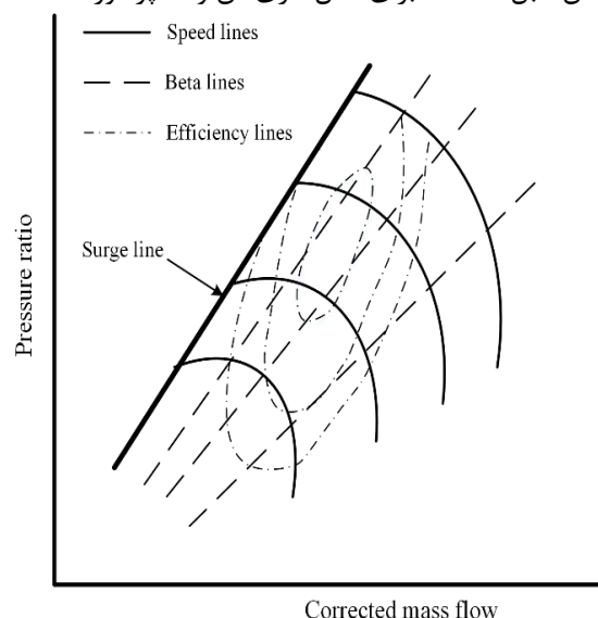
شکل (۴): نمای کلی نقشه عملکردی یک کمپرسور
