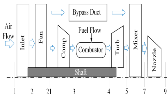
شکل (۱): شماتیک اجزای موتور میکرو-توربوفن با جریان آمیخته
