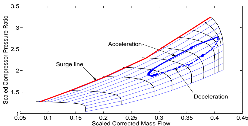
شکل (۱۷): نمایش مسیر شتاب‌گیری موتور روی نقشه عملکردی کمپرسور
