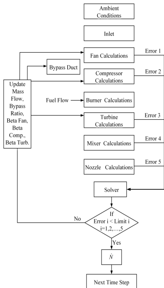
شکل (۵): روش تکرار ماتریسی برای مدل سازی ترمودینامیکی موتور
