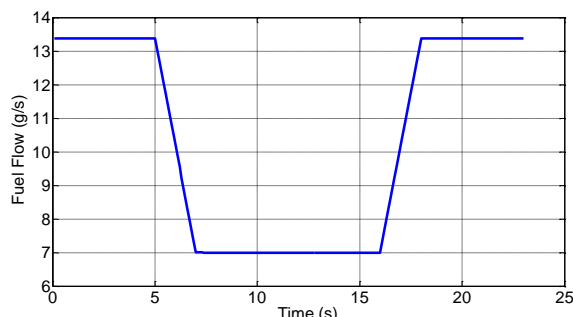
شکل (۱۵): برنامه سوخت موتور برای تحلیل عملکرد گذرا
