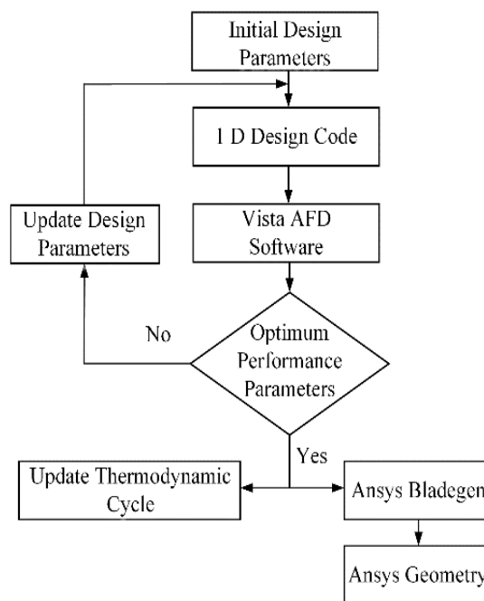
شکل (۷): روند طراحی اولیه فن
