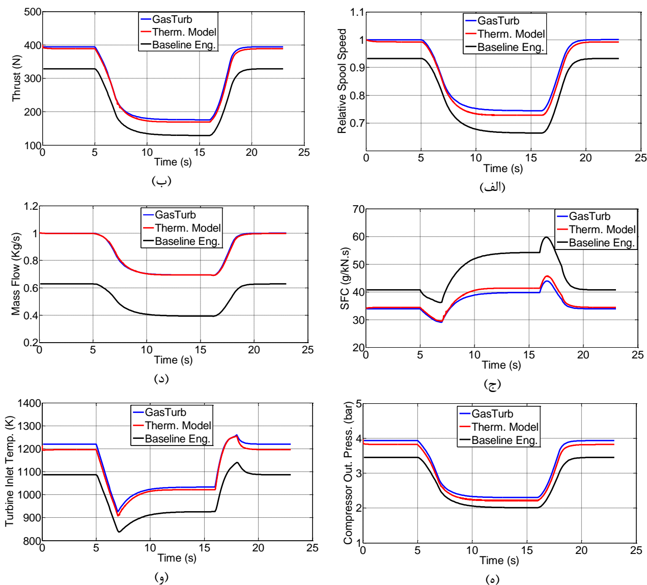
شکل (۱۶): عملکرد موتور میکرو-توربوفن در سناریوی گذرا: الف) سرعت نسبی شفت، ب) تراست، ج) مصرف سوخت ویژه، د) دبی هوای ورودی، ه) فشار خروجی کمپرسور، و) دمای ورودی توربین
