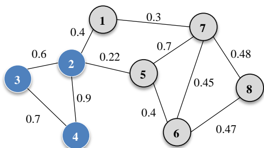
شکل ۱۲. خوشه‌های نهایی در گراف وزن دار اولیه
