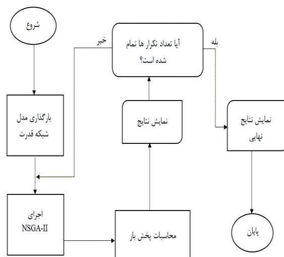
شکل ۹. ساختار روش NSGA-II
