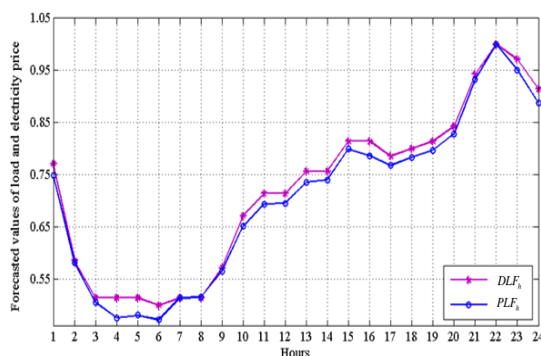
شکل ۱۱. نمودار درخواست توان و قیمت برق برای یک شبانه‌روز
