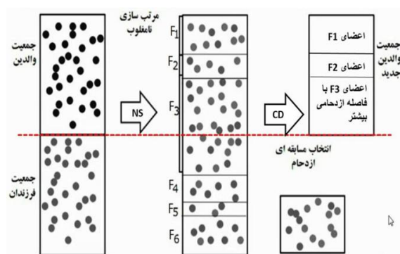
شکل ۳. انتخاب نسل جدید در NSGA-II
