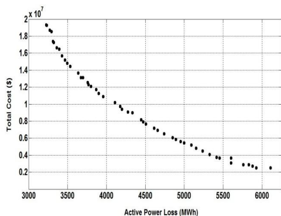
شکل ۱۱. نمودار جبهه پارتو سامانه ۳۳ باسه
