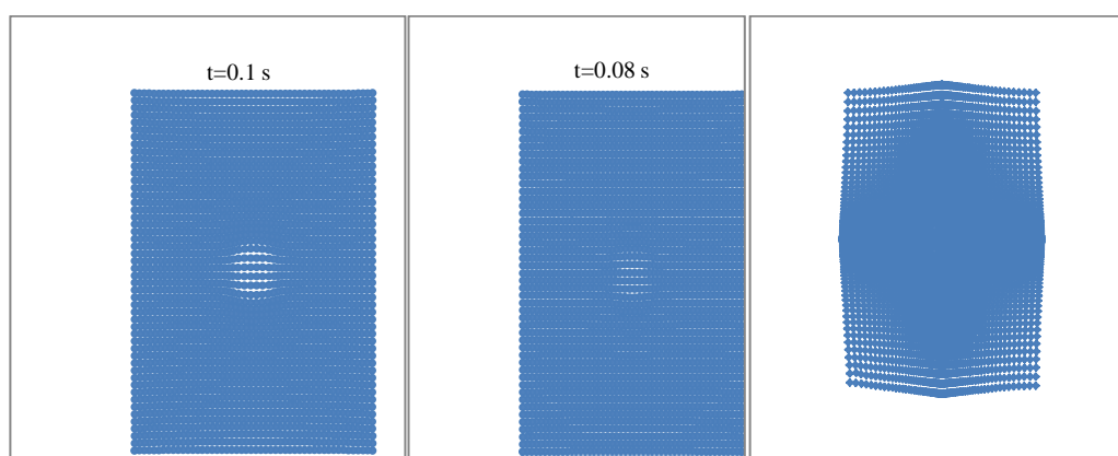
شکل ۵. تشکیل حباب انفجار در زمان های متفاوت
