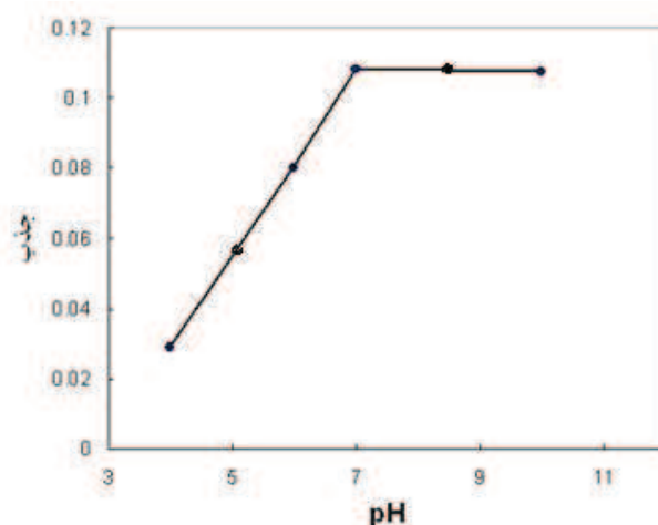
شکل ۳. اثر pH بر جذب کمپلکس اورانیل برم پاداپ، غلظت ۰/۵ ppm، بافرهای تری اتانول آمین و فسفات و ۳ میلی لیتر EDTA ۰/۰۱ مولار
