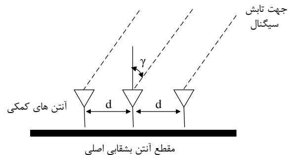
شکل (۴). چیدمان آنتن‌های اصلی و کمکی نسبت به یکدیگر
