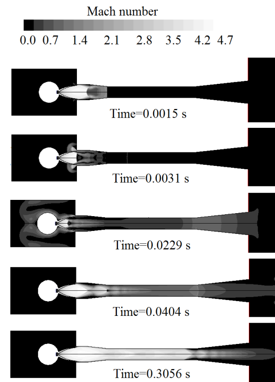
شکل (۱۶): کانتور عدد ماخ جریان در زمان های مختلف بعد از محو شدن دیافراگم.
