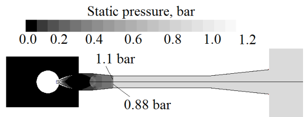
شکل (۱۵): کانتور فشار استاتیک جریان در پشت دیافراگم در لحظه محو شدن دیافراگم.
