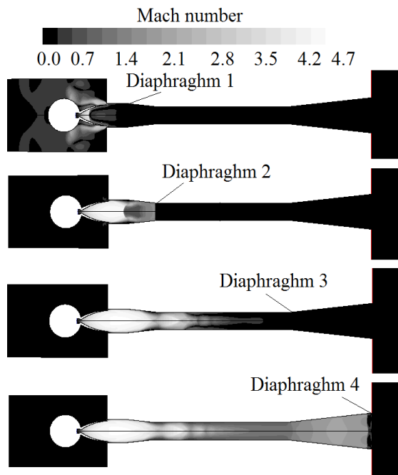
شکل (۱۸): کانتور عدد ماخ جریان در لحظه ماقبل محو شدن دیافراگم در موقعیت‌های مختلف دیافراگم
