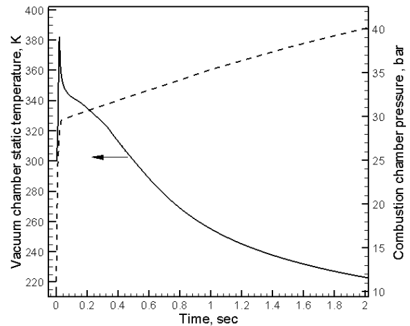
شکل (۱۲): دمای استاتیک متوسط سیال در محفظه خلاء برحسب زمان در حالت بدون پیش خلاء.
