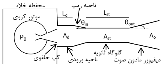
شکل (۱): شماتیکی از اجزای اصلی یک تستند خلاء
